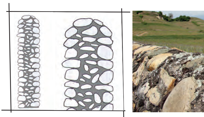
Mur en galets avec couronnement en galets visibles
