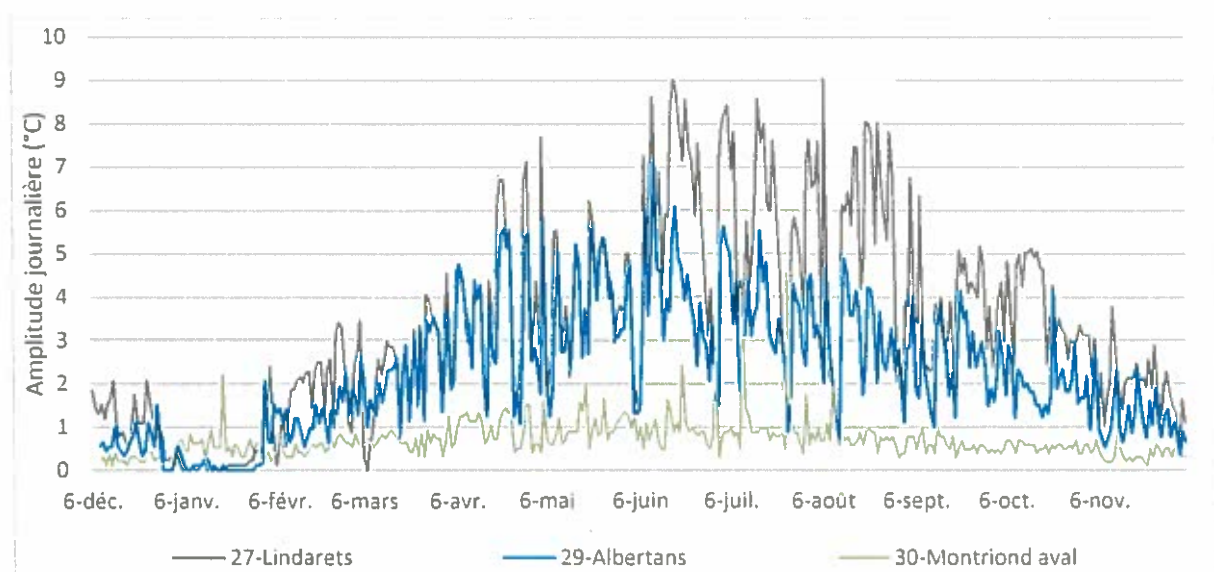
Figure 1 Amplitudes journalières sur les trois stations de la Dranse de Montriond
