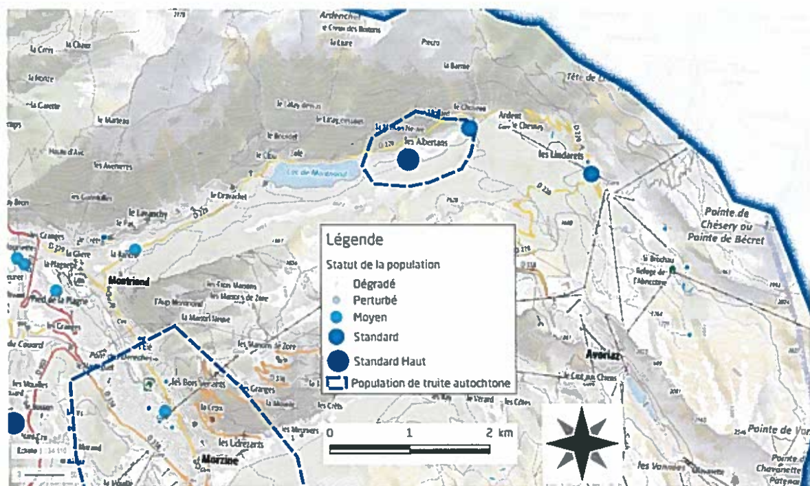
Figure 3. Statut des populations de truite des quatre stations de la Dranse de Montriond par rapport au standard départemental des DENSITÉS
