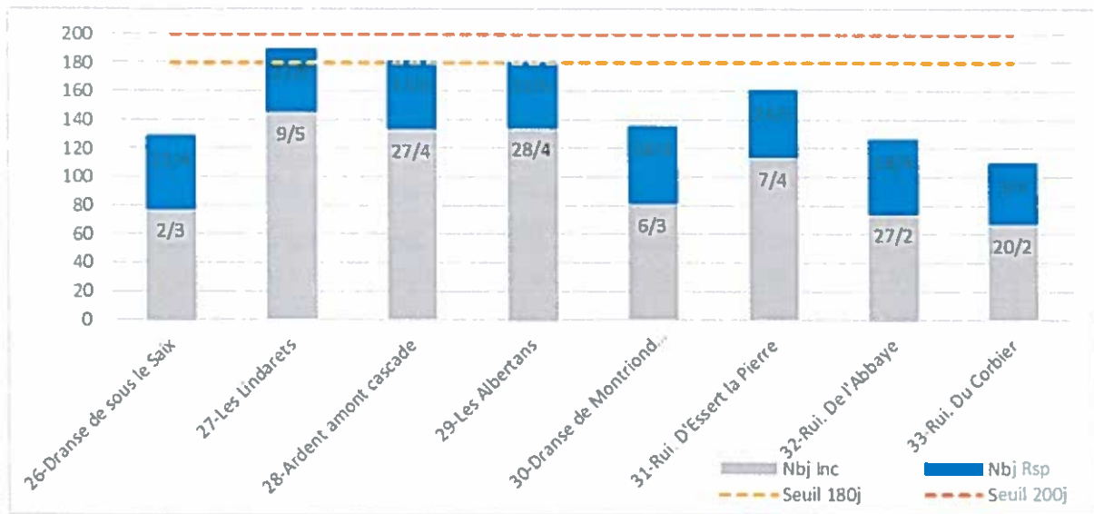
Figure 2 : Nombre de jours de la phase d'incubation des œufs (NbJ Inc), de la phase de résorption (NbJ Rsp) et seuils des 180 jours et 200 jours pour les stations des affluents rive droite. Les dates correspondent aux dates d'éclosion (D50 Ecl, en bas) et d'émergence de 50% des alevins (D50 Emg, en haut).
