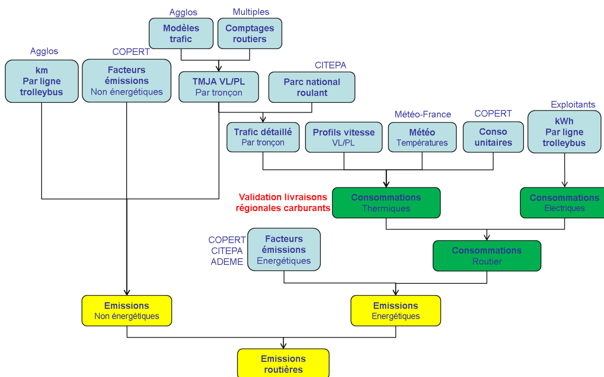
Figure 11 : Chaîne de calcul simplifiée des émissions du transport routier
