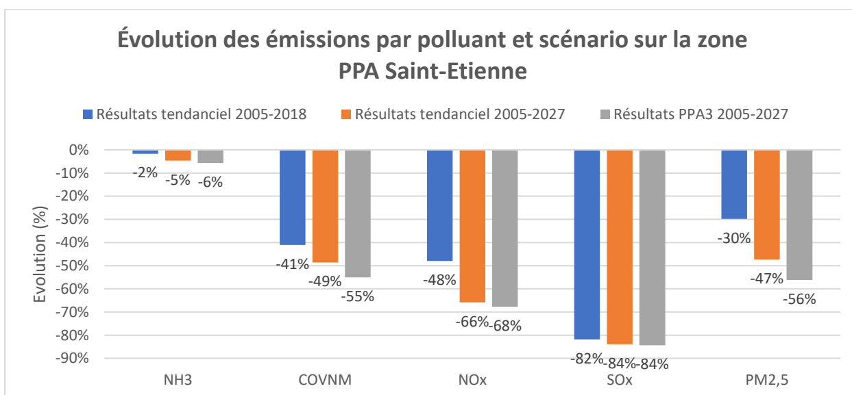
Figure 61 - Évolution des émissions par polluant et scénario sur la zone PPA Saint-Etienne
