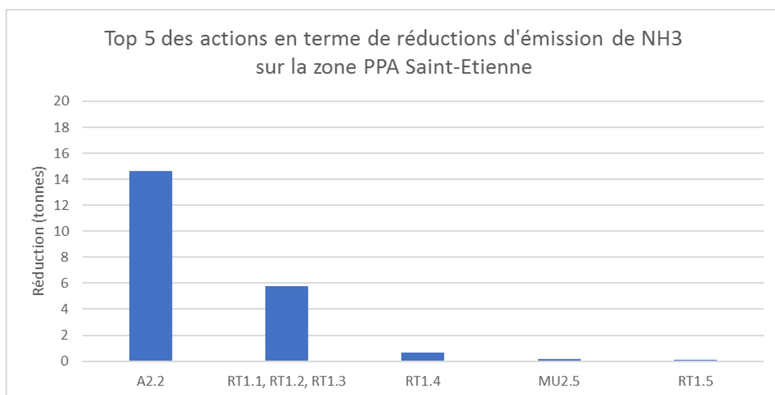
Figure 84 - Top 5 des actions en termes de réductions d'émission de NH3 sur la zone PPA Saint-Etienne
