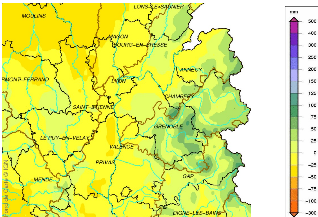
Cumul de pluies efficaces— Avril 2017
