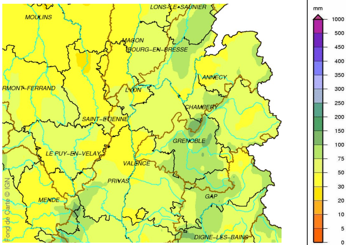
Cumul de précipitations— Avril 2017
