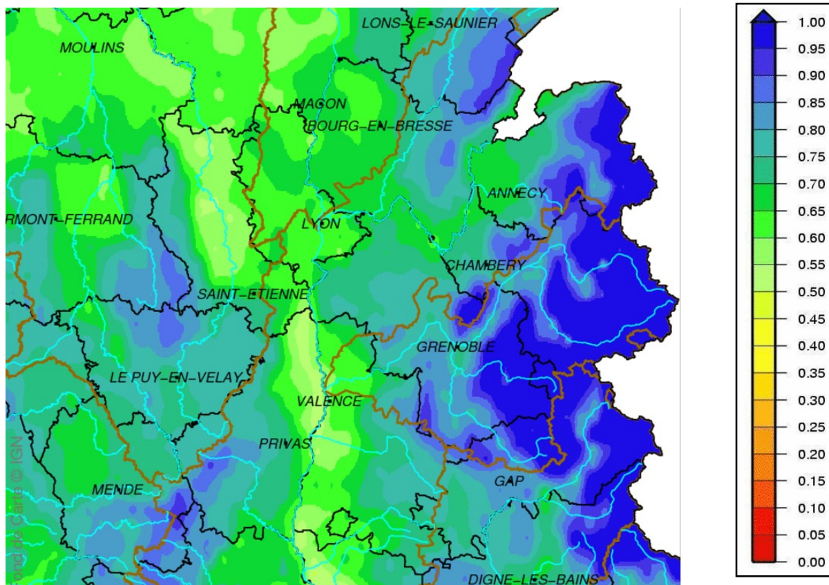
Indice d'humidité des sols au 1 er mai 2017
