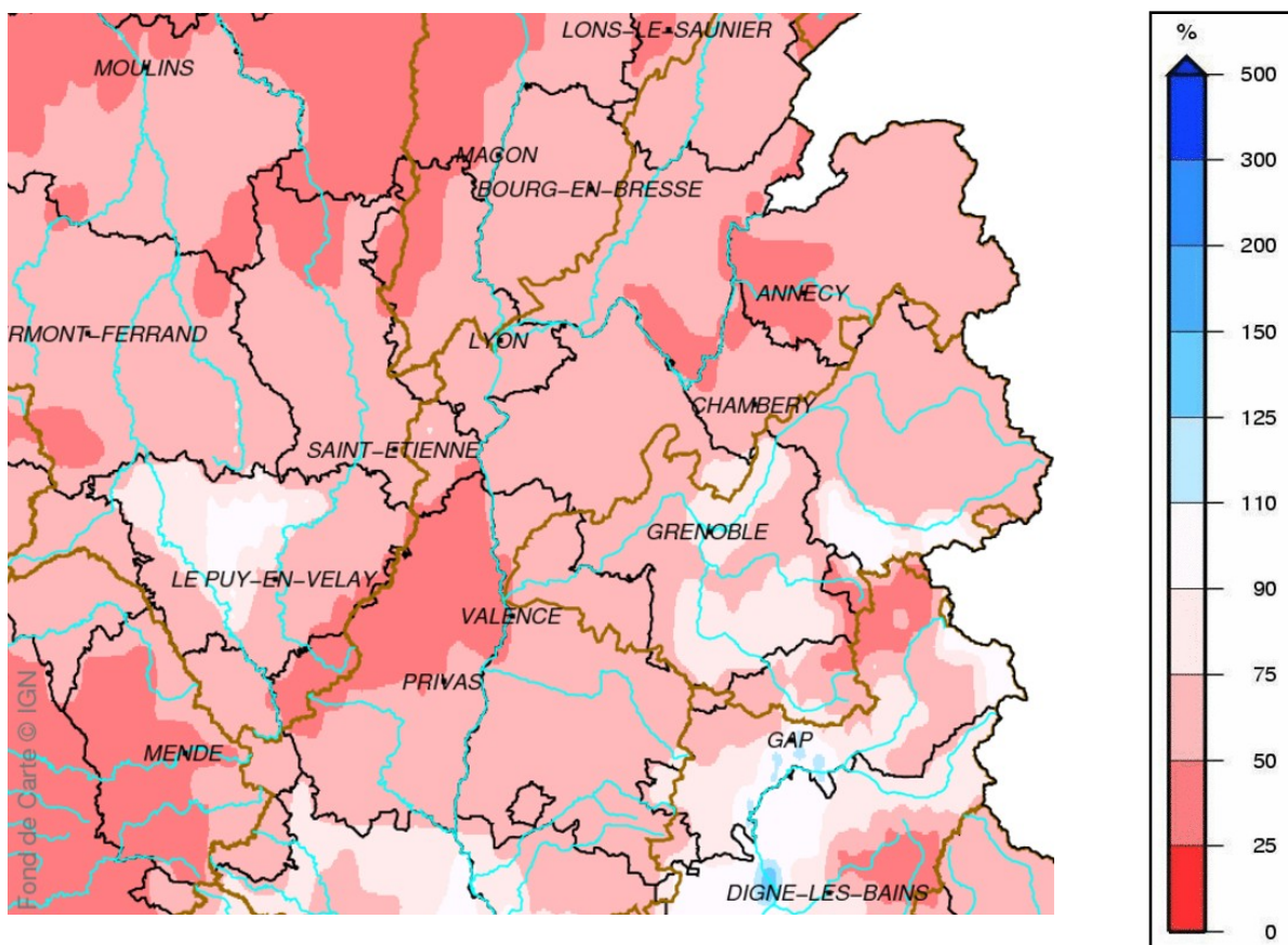
Rapport à la normale 1981-2010 des précipitations— Avril 2017
