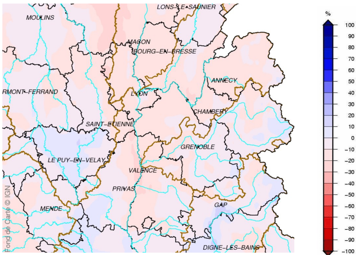
Écart pondéré à la normale 1981-2010 de l'indice d'humidité des sols au 1 er mai 2017
