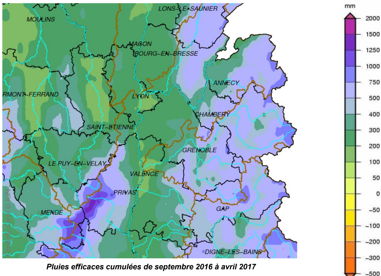
Cumul de pluies efficaces— Avril 2017
