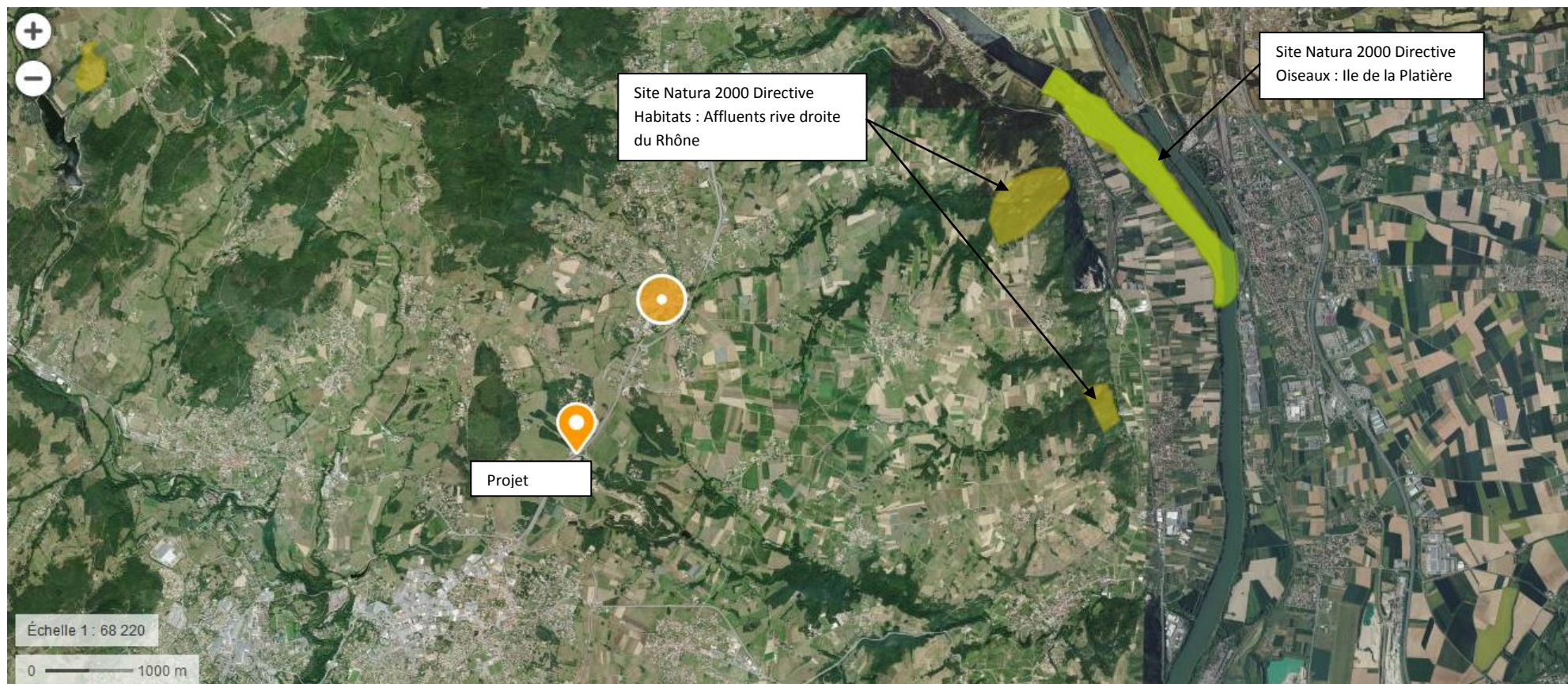
Figure 1 : Localisation sur photo aérienne au 1/68220 de la localisation des sites Natura 2000 les plus proches (photo aérienne de 2016)
