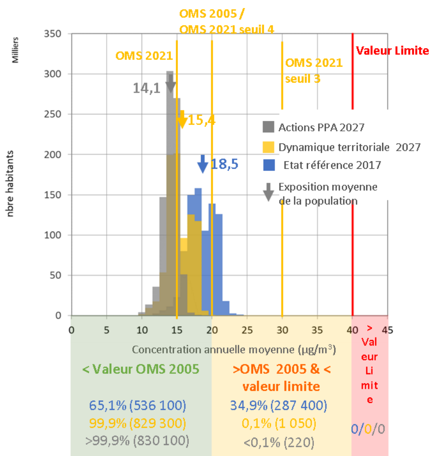
Figure 88 : Histogramme de distribution de l'exposition de la population aux particules PM10 selon l'état de référence (bleu), le scénario « Dynamique territoriale » 2027 (jaune), et le scénario Actions PPA 2027 (gris)
