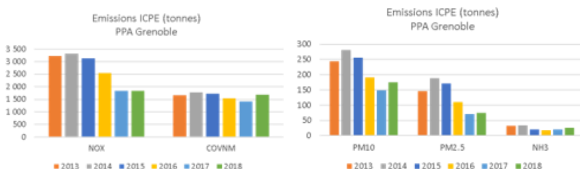
Figure 57 : Evolution des émissions des ICPE entre 2013 et 2018 sur le territoire PPA pour aider à fixer les hypothèses d'évolution 2018-2027 des émissions
