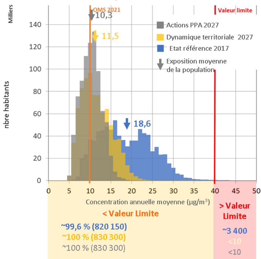
Figure 74 : Histogramme de distribution de l'exposition de la population au dioxyde d'azote selon l'état de référence (bleu), le scénario « Dynamique Territoriale » 2027 (jaune), et le scénario Actions PPA 2027 (gris)
