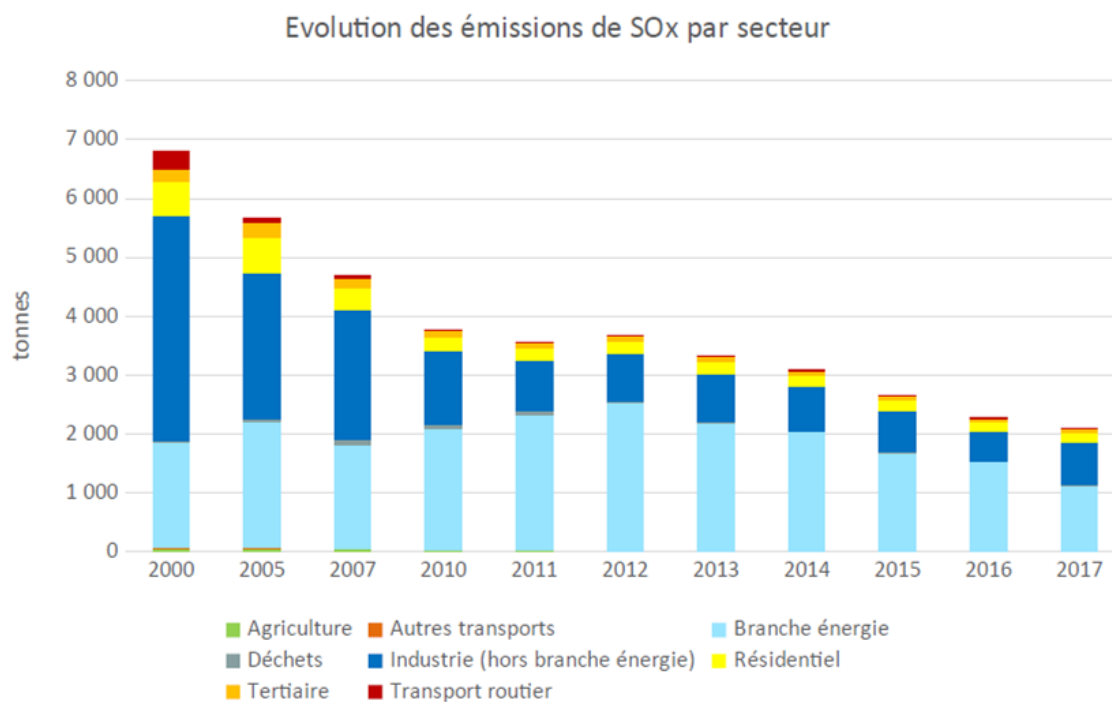
Figure 25 : Evolution des émissions de SOx par secteur sur le périmètre d'étude du PPA
