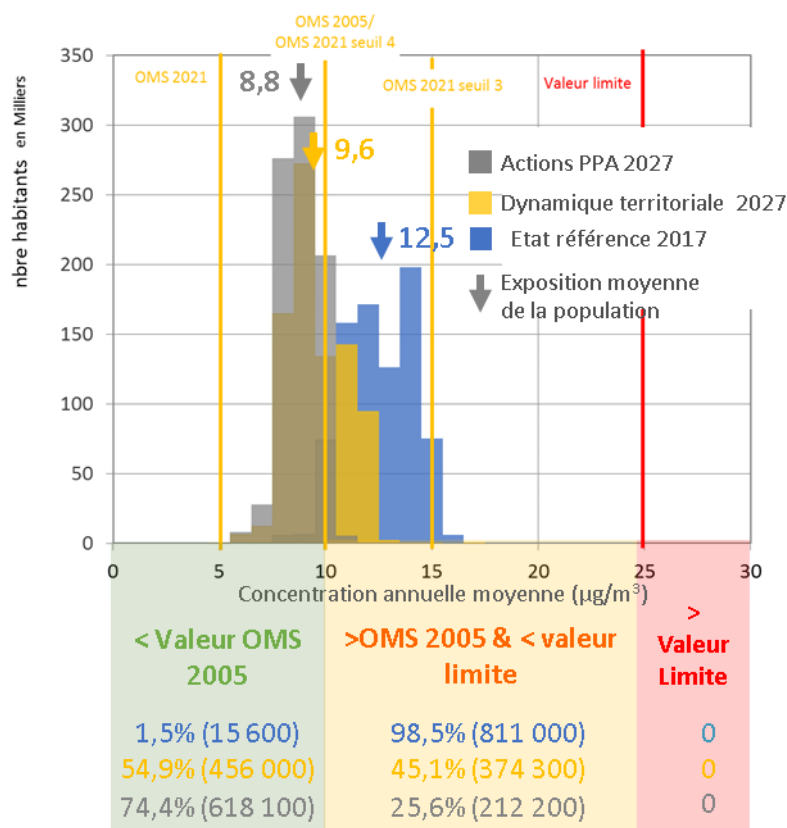
Figure 81 : Histogramme de distribution de l'exposition de la population aux particules PM2.5 selon l'état de référence (bleu), le scénario Dynamique territoriale 2027 (jaune), et le scénario Actions PPA 2027 (gris)
