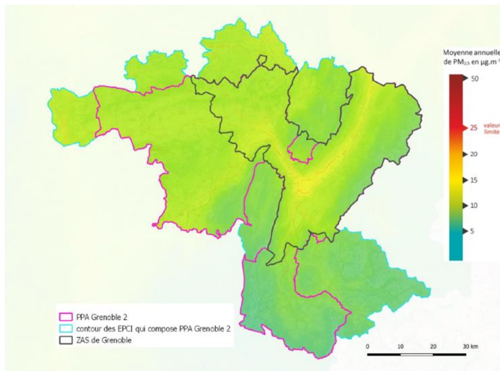
Figure 37 : Concentrations annuelles en PM 2,5 en 2017
