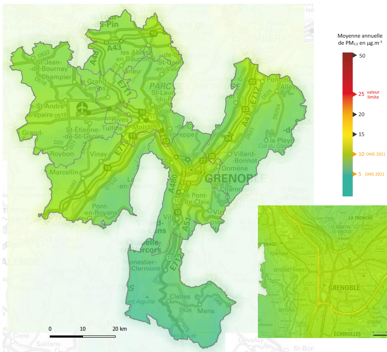
Figure 78 : Cartographies des concentrations moyennes annuelles en PM 2.5 attendues selon le scénario Actions PPA 2027
