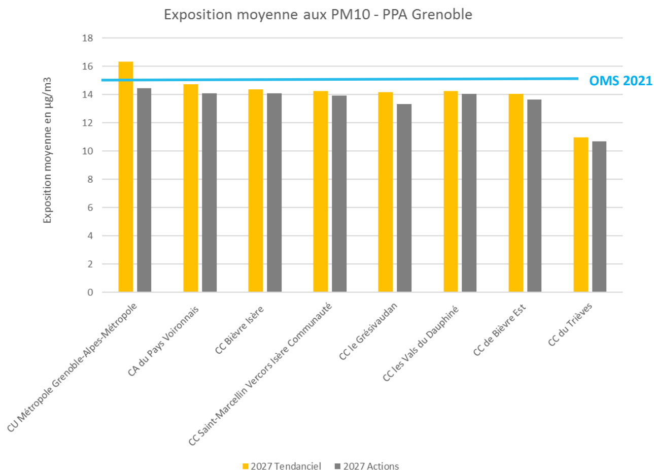
Figure 89 : Evolution de l'exposition moyenne au PM10 sur le périmètre PPA entre le scénario « Dynamique territoriale » 2027 et Actions 2027
