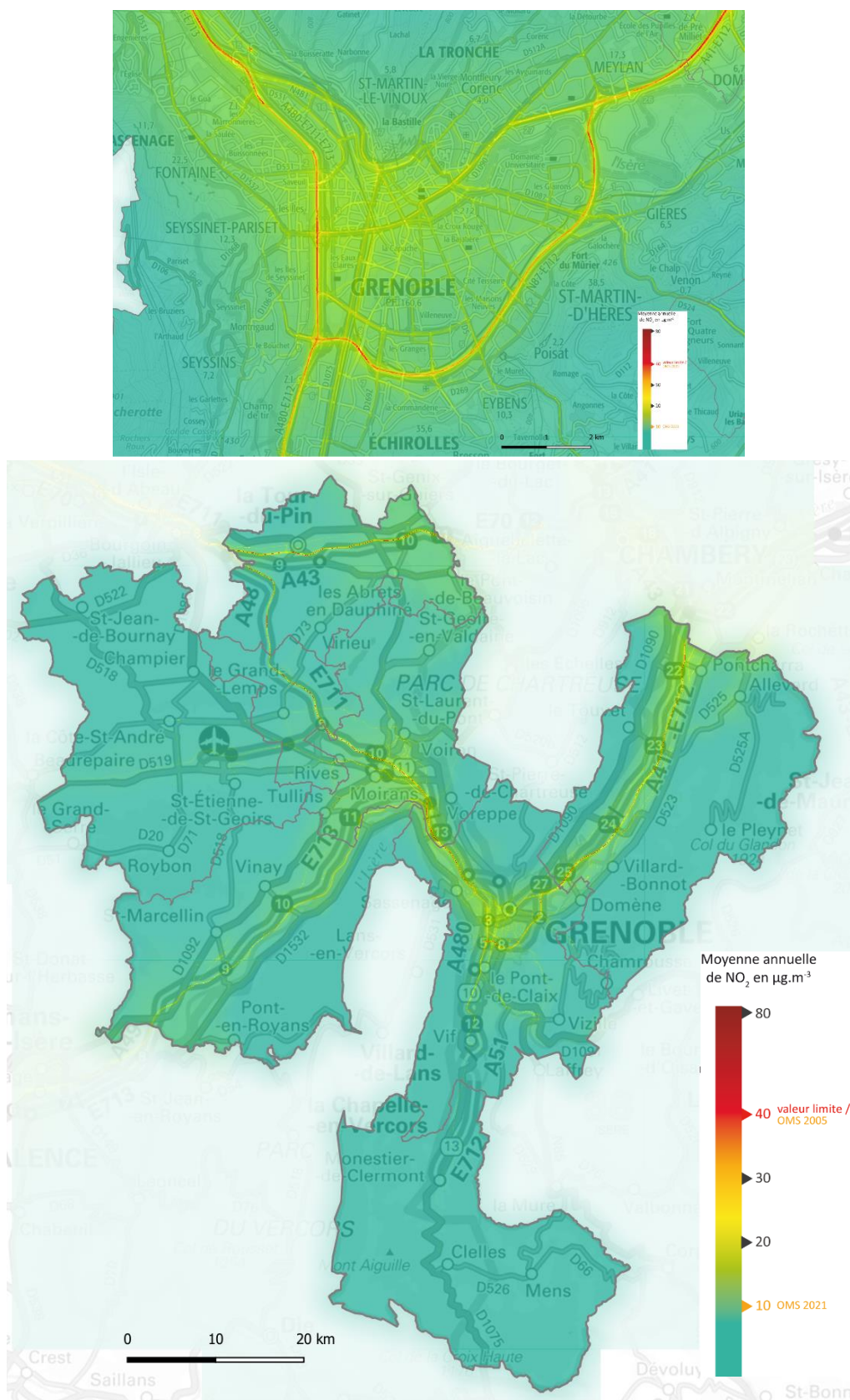
Figure 71 : Cartographies des concentrations moyennes annuelles en \text{NO}_2 attendues selon le scénario Actions PPA 2027
