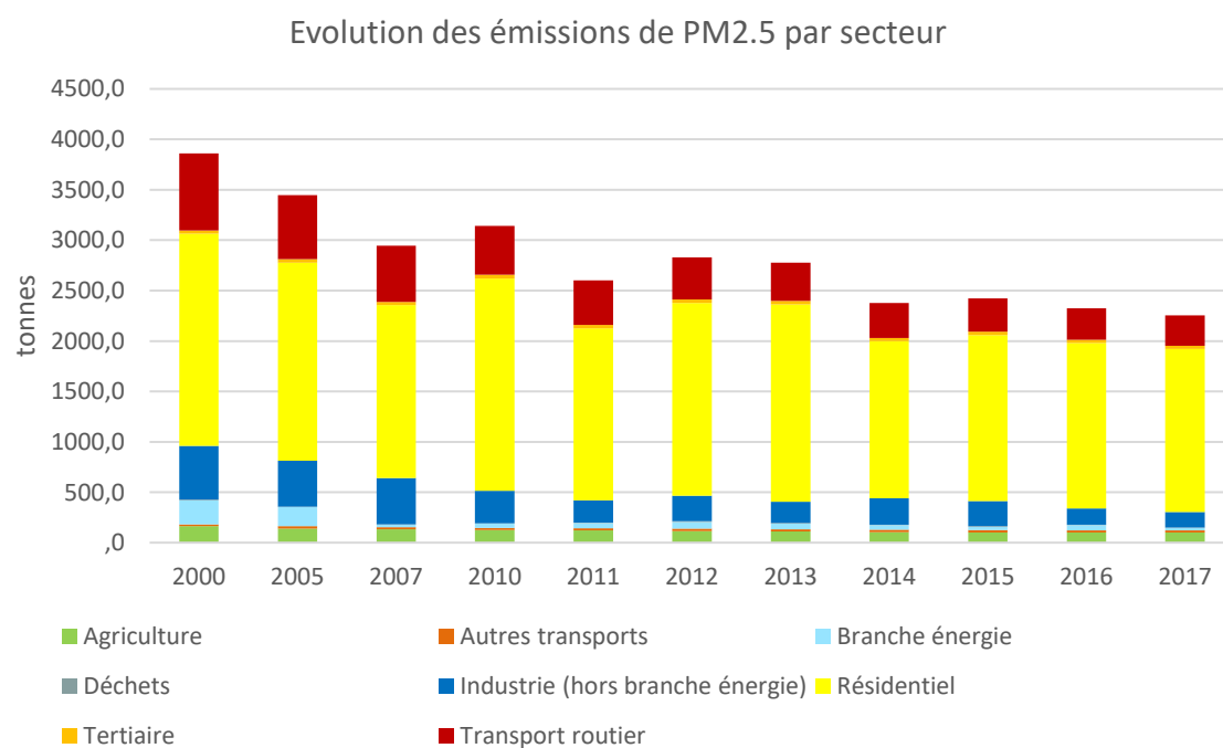
Figure 22 : Evolution des émissions de PM 10 et PM 2.5 par secteur sur le périmètre d'étude du PPA
