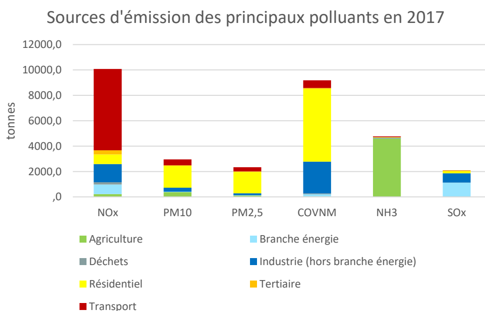
Figure 19 Quantité et origine des émissions des principaux polluants
