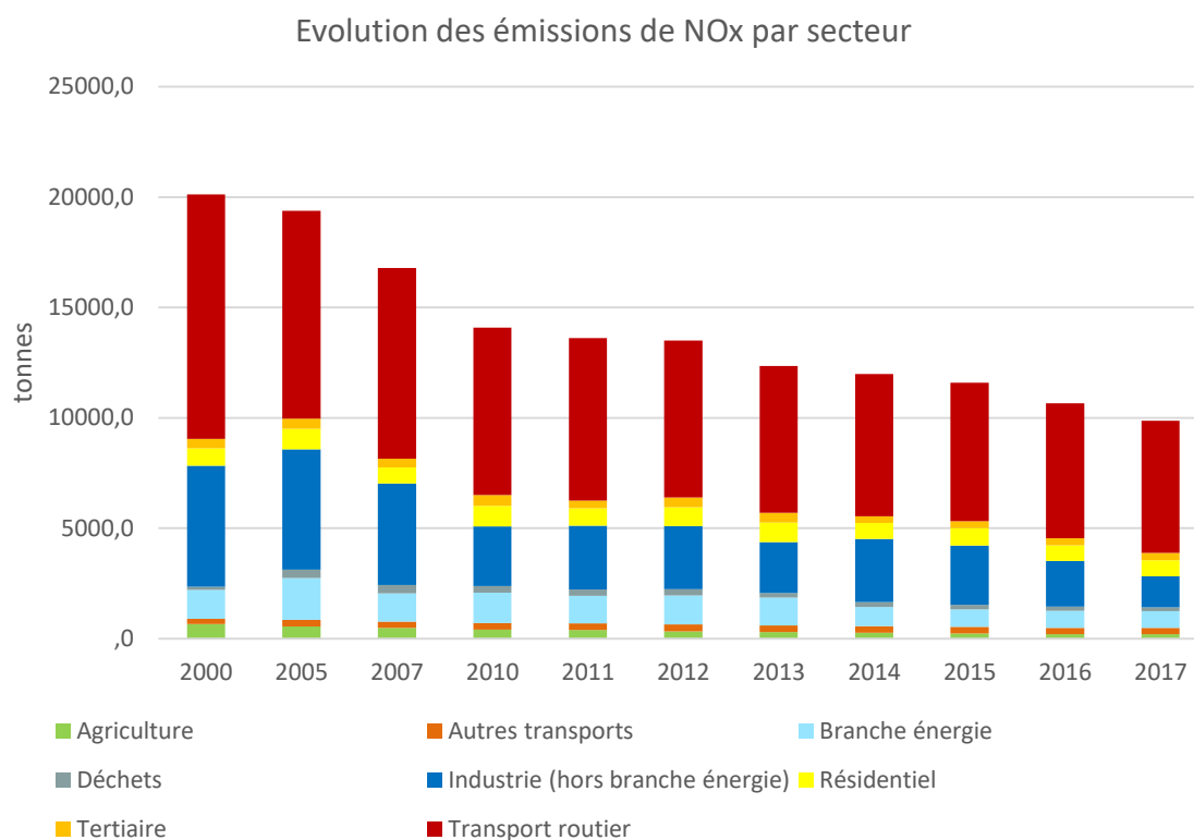
Figure 21 : Evolution des émissions de NOx par secteur sur le périmètre d'étude du PPA
