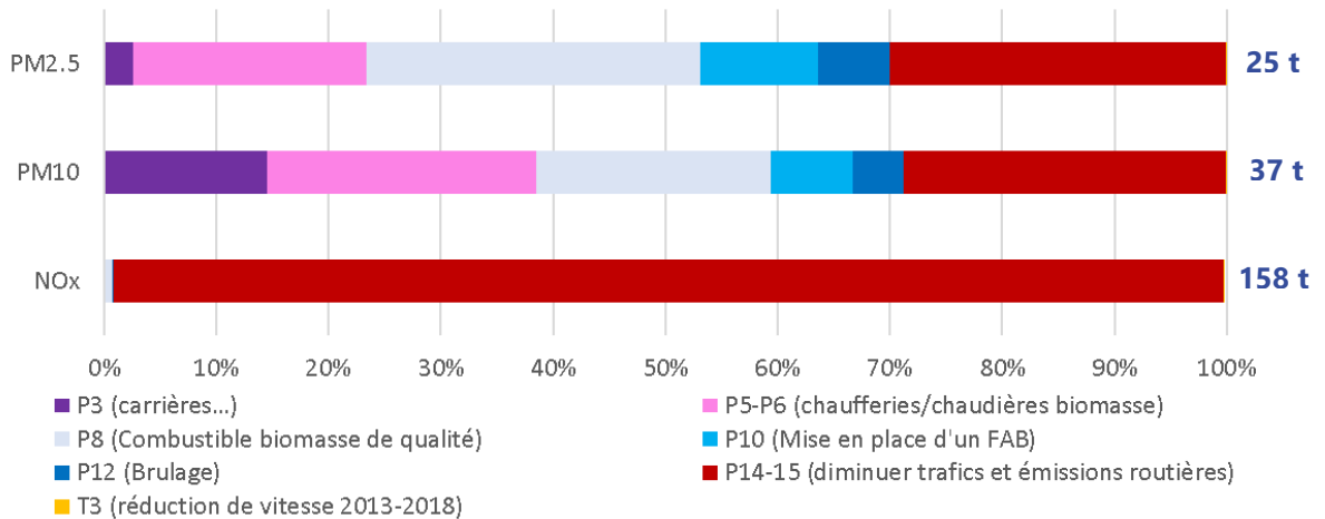
Figure 54 : répartition des gains en émissions par action du PPA – PPA Lyon
