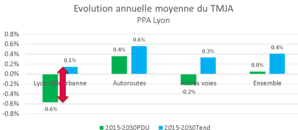
Figure 47 : évolution annuelle moyenne du TMJA entre 2015 et 2030 selon deux projections trafics
