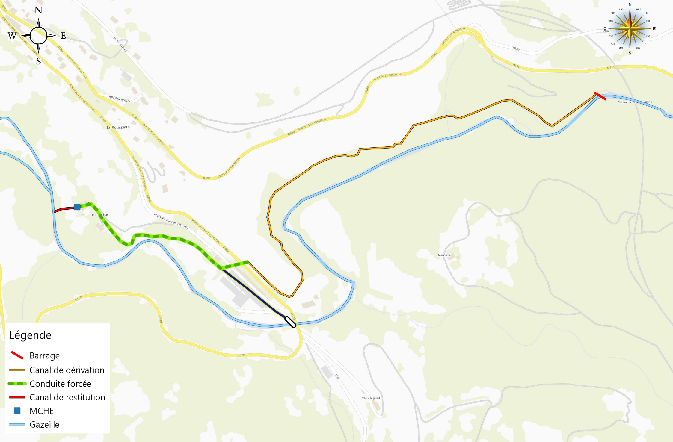
Plan du projet de la MCHE du Moulin d'Arcis - 1/5 000
