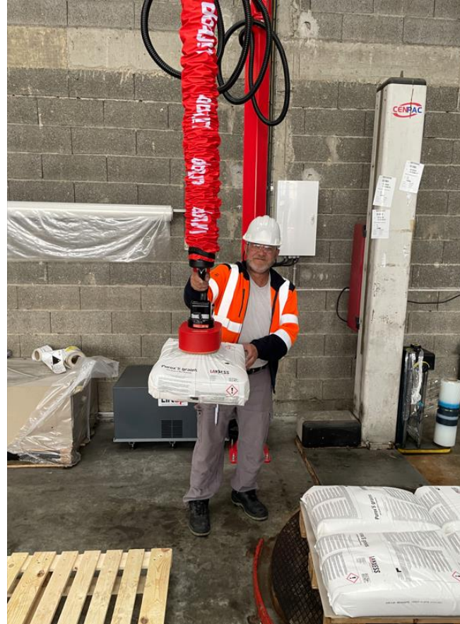
Préhenseur
