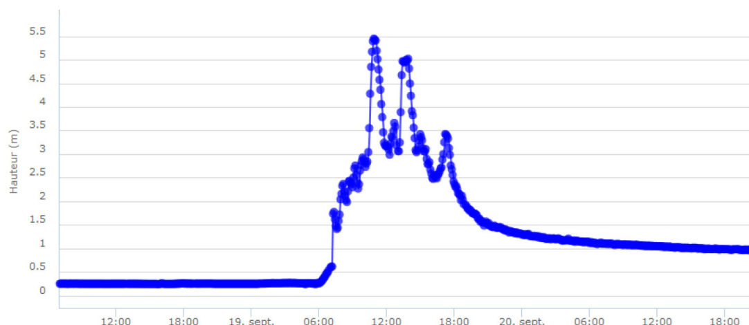
Diagramme de crue de l'Hérault à Valleraugue (30) (diagramme extrait du rapport REX rapide - Crue du 19 septembre 2020 sur l'Hérault du service de prévision des crues (SPC) Méditerranée Ouest du 22/09/2020)
