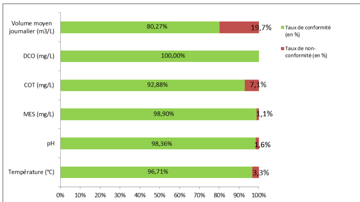
Figure 4 : Taux de conformité aux VLE des paramètres suivis quotidiennement dans les rejets aqueux en 2021
