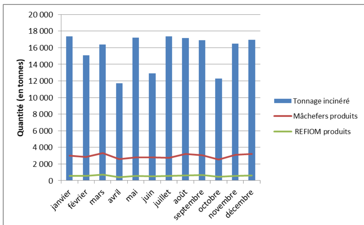
Figure 11 : Évolution des quantités de mâchefers et de REFIOM produits en 2020 en fonction des quantités incinérées
