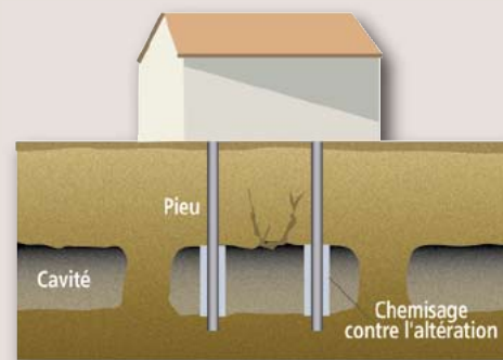
Les fondations profondes
