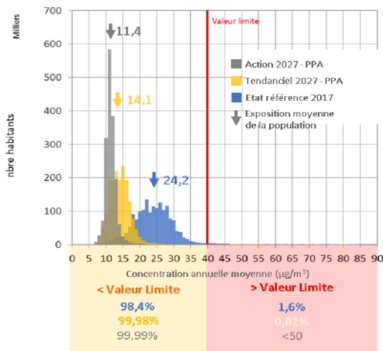
Figure n°43. Distribution de l'exposition de la population au NO 2 - scénario tendancier 2027/Action 2027 (source : ATMO AURA)
