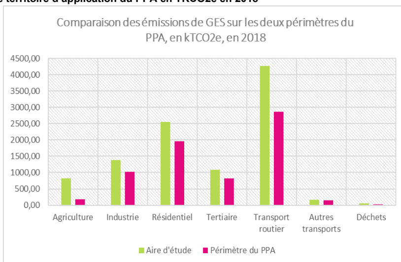
Figure n°34. Emissions de GES par secteur sur le territoire d'application du PPA en TKCO2e en 2018
