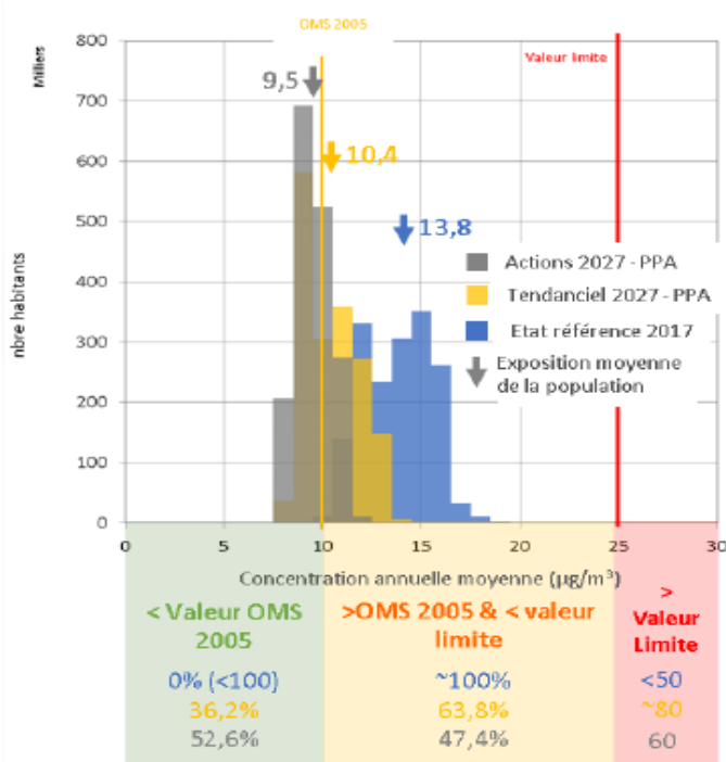
Figure n°44. Distribution de l'exposition de la population aux PM2.5 - scénario tendanciel 2027/Action 2027 (source : ATMO AURA)
