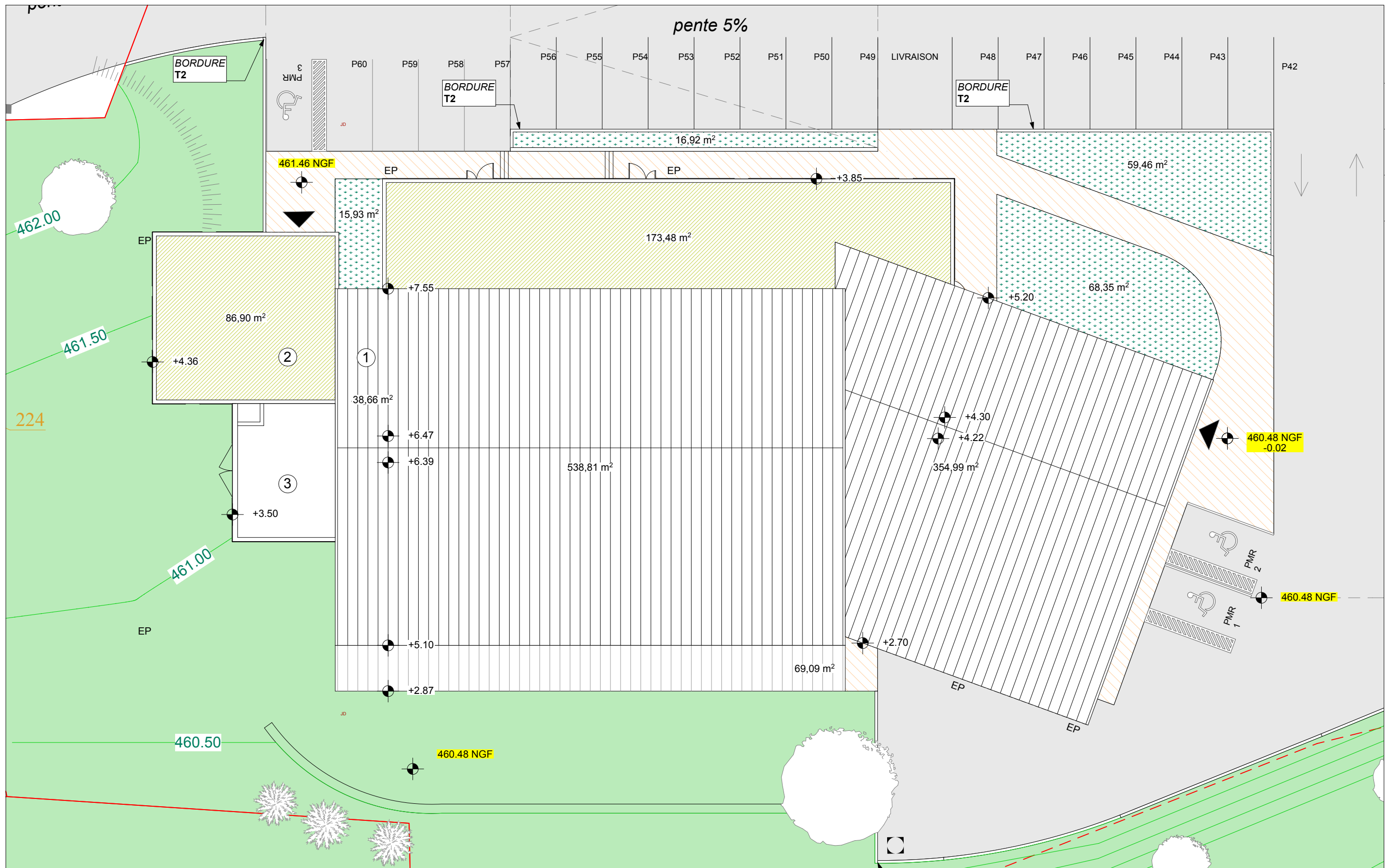
5 - TOITURES - ech. 1/200
